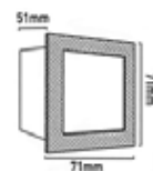
71989 EN860-9907WH IP54-0.8W 9LEDs H.51mm L.71mm I.71mm
