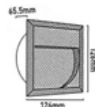
71984 EN860-9903WH IP65-1.2W 14LEDs H.65.5mm L.120mm I.126mm
